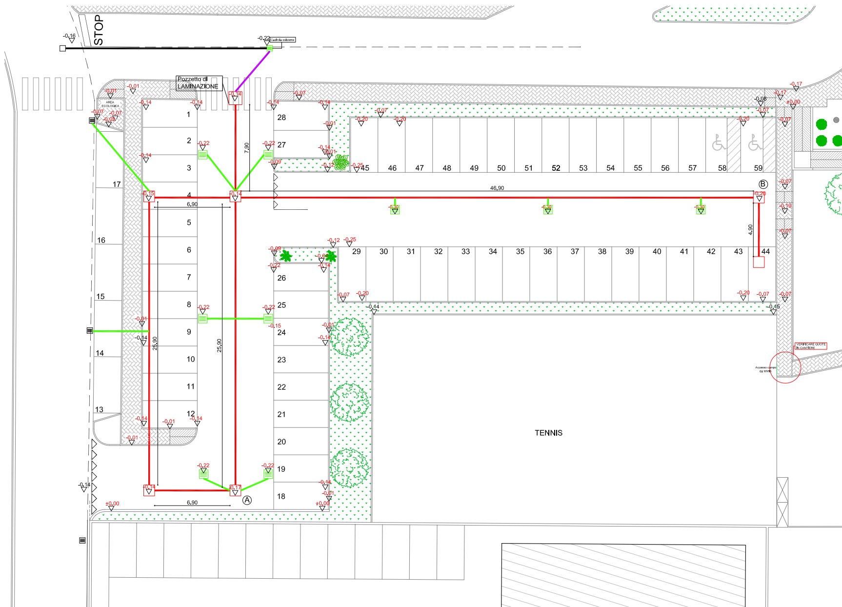
PIANTA PARCHEGGIO - STATO DI PROGETTO
